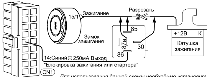
Схема 10. Для использования данной схемы необходимо установить значение 1 (заводское значение) программируемой функции 22
