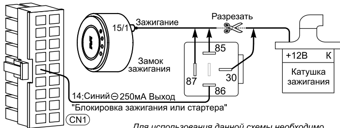
Схема 11. Для использования данной схемы необходимо установить значение 2 программируемой функции 22
